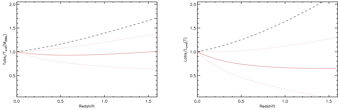
FIGURE 7.20 – Evolutions des lois d’échelle T-M_{200c} et L-T prédites par le « meilleur modèle » et décrites par les Eq. 6.10 et 6.11. La ligne rouge pleine indique l’évolution prédite pour le meilleur modèle ( \Omega_m = 0,24 , \gamma_{z,MT} = 0,8 et \gamma_{z,LT} = -1,3 ), les lignes en pointillés délimitant la zone de confiance à 68%. La ligne discontinue noire montre l’évolution attendue dans le cas auto-similaire ( \gamma_{z,MT} = \gamma_{z,LT} = 0 ).
