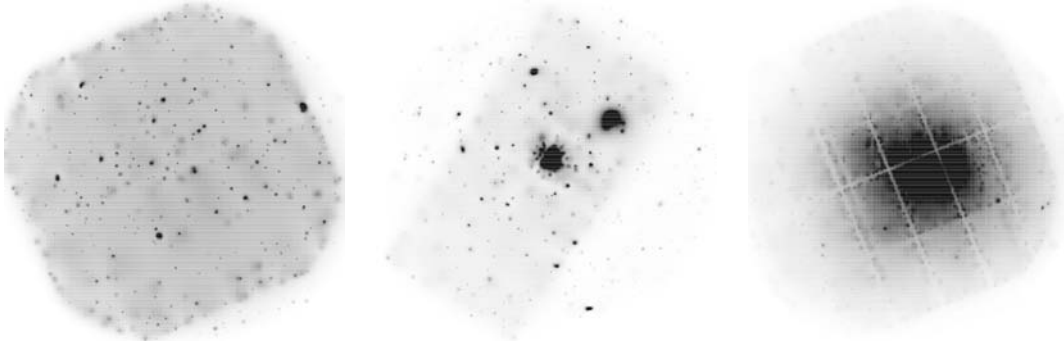
FIGURE 5.7 – Trois exemples de pointés éliminés de l’analyse cosmologique. Gauche : l’observation est affectée par de longues périodes de flares qui n’ont pas pu être reitrés par la procédure de préfiltrage automatique (ObsId : 0039140101). Centre : le détecteur PN est en mode Large Window et seules ses CCD centrales collectent des photons (ObsId : 0083150401). Droite : observation de l’amas Coma, source très étendue empêchant la détection de sources d’arrière-plan (ObsId : 0300530301).
