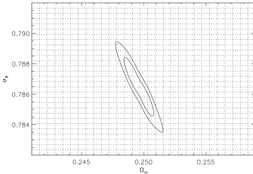
FIGURE 6.11 – Exemple de calcul de vraisemblance (Eq. 6.25) sur une grille de 30 \times 30 valeurs pour \Omega_m et \sigma_8 . Les contours montrés ici contiennent 68% et 95% de la vraisemblance (équivalant à des niveaux de confiance de 1 et 2 \sigma respectivement). Si l'on désire rajouter un paramètre dans l'étude, il faut multiplier le temps de calcul par un facteur 30, et ainsi de suite, ce qui rend la méthode fastidieuse.
